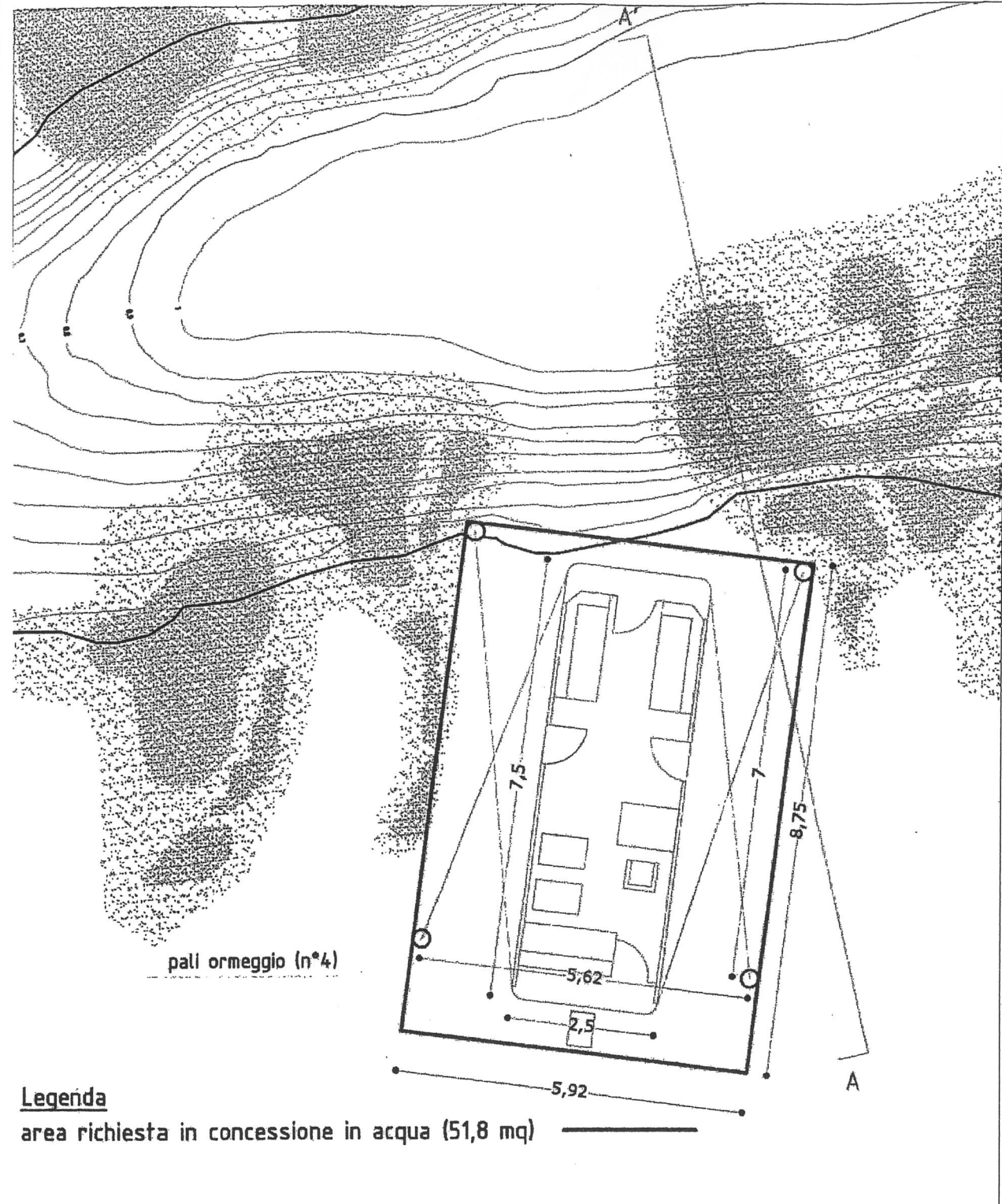
Planimetria scala 1:100
