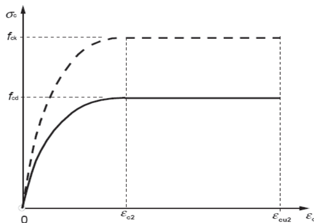
Legame costitutivo di progetto parabolotta-rettangolo per il calcestruzzo.
