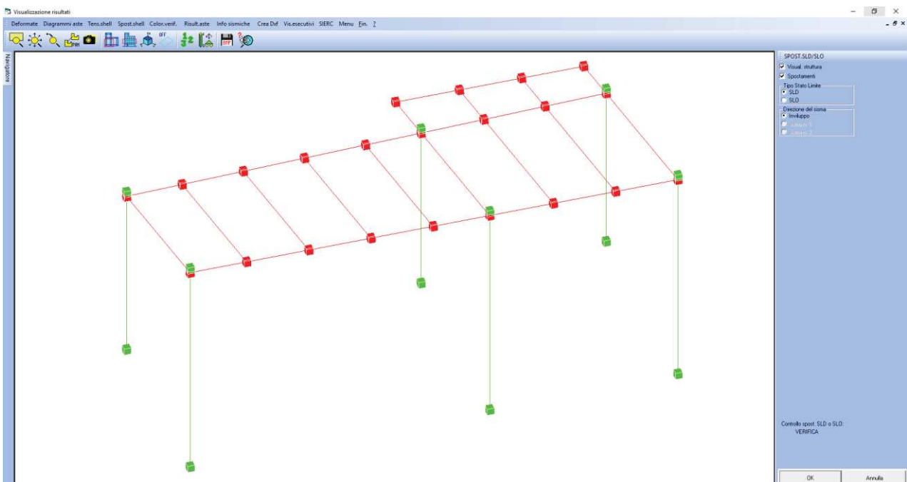
Figura 1 - Verifica spostamenti SLD
