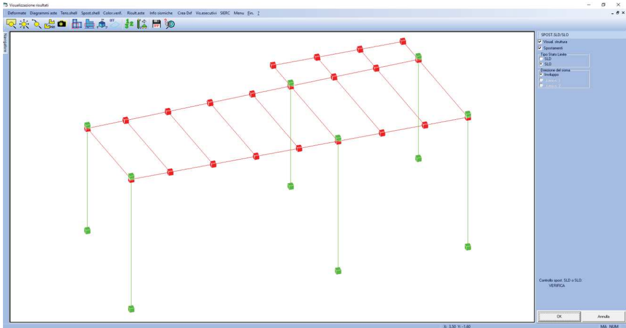
Figura 2 - Verifica spostamenti SLO
