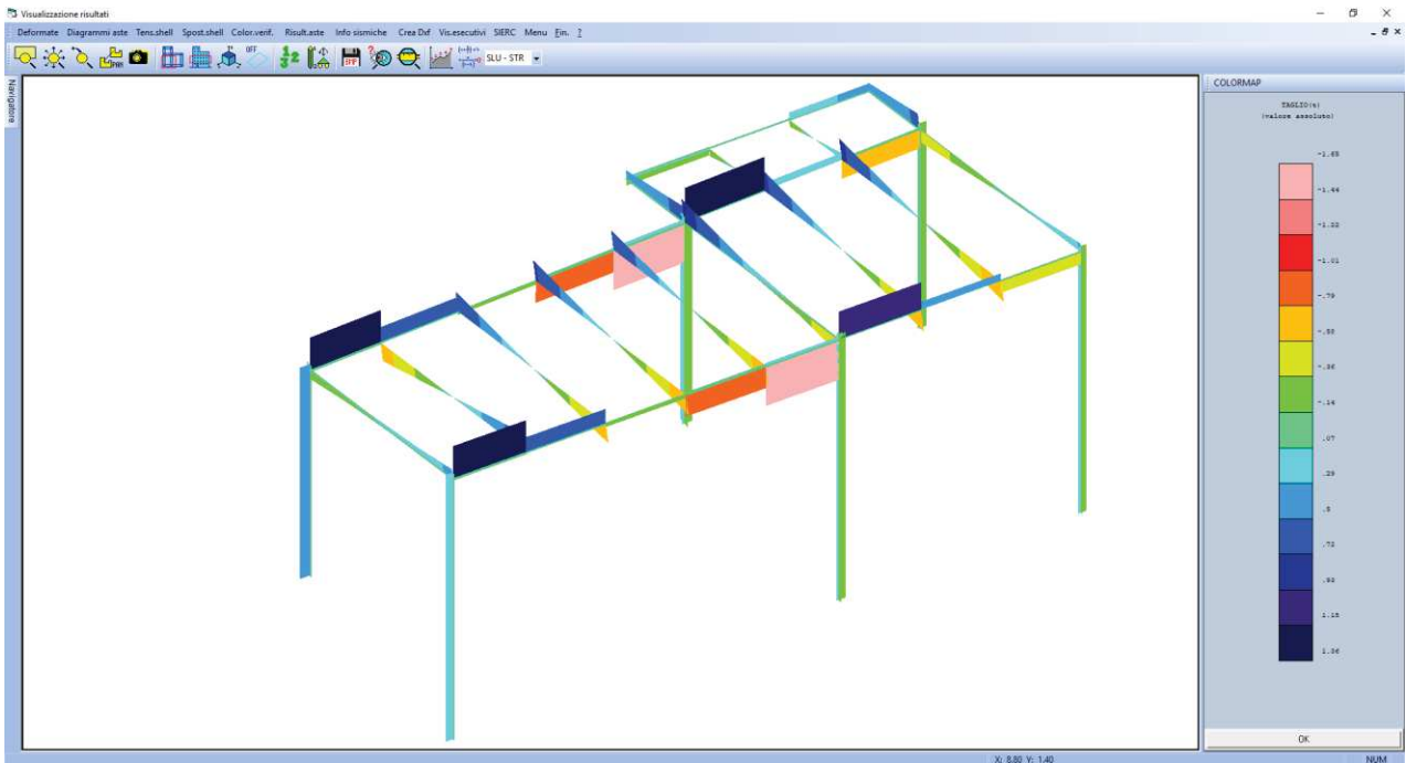
Figura 5 - Diagramma taglio
