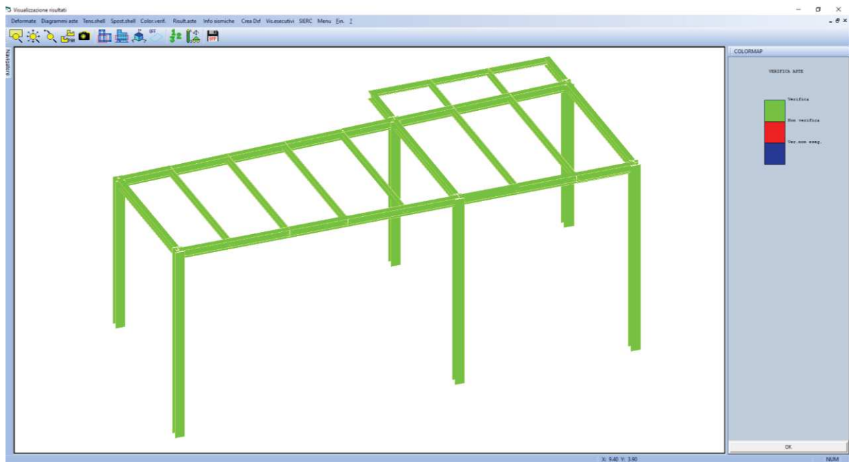
Figura 3 – Aste verificate
