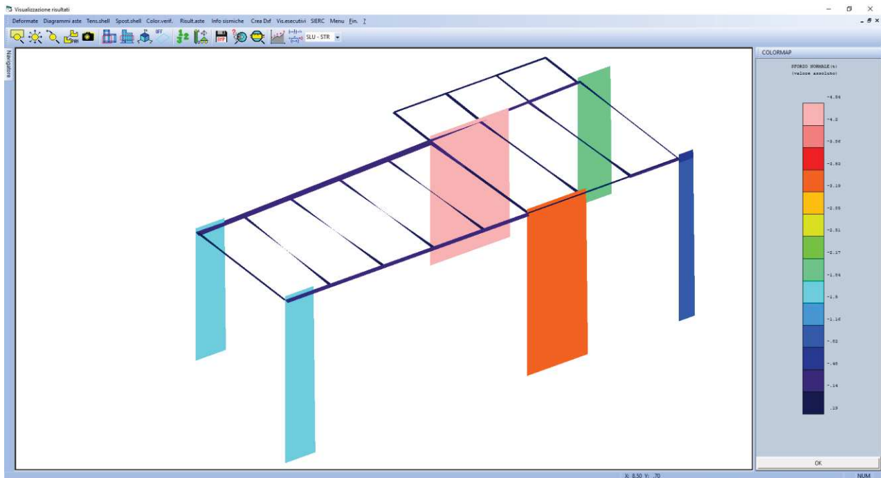
Figura 6 - Diagramma Sforzo Normale
