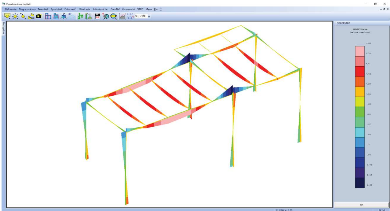
Figura 4 - Diagrammi momento flettente
