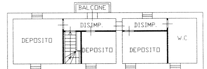
PIANTA PIANO PRIMO H= 3.25
